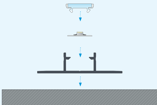
PL Instrukcja montażu profilu NIPO z kloszem TERRA.
