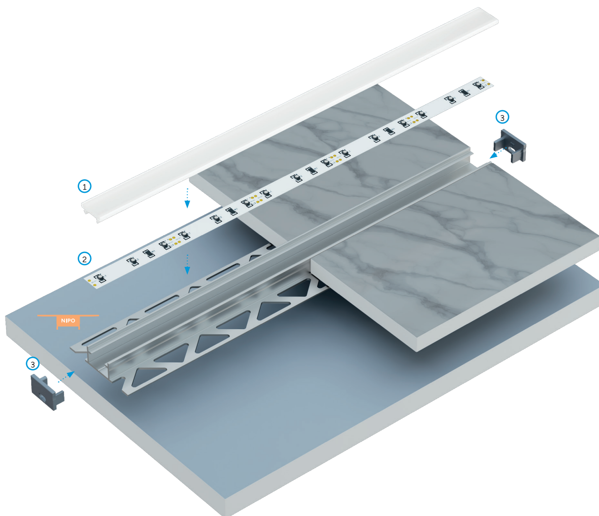
PL Schemat złożenia elementów systemu oświetleniowego z wykorzystaniem profilu NIPO oraz (1) klosza TERRA, (2) taśmy LED, (3) oraz zaślepek z otworem.
