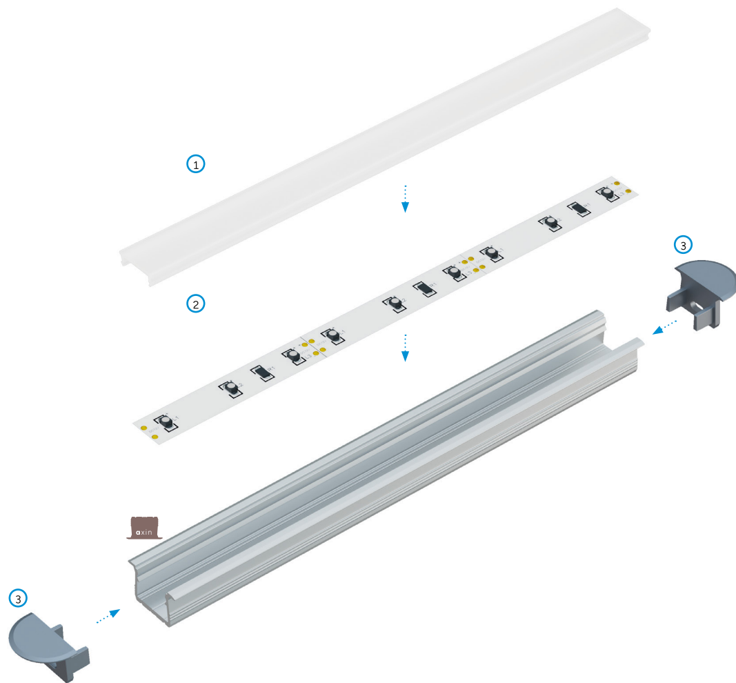
Montageplan für Elemente des LED-Beleuchtungssystems mit axin LED-Profil und (1) Nano-Abdeckung , (2) LED-Streifen , (3) Endkappen mit Löchern .
