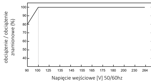
CHARAKTERYSTYKA OBCIĄŻALNOŚCI W ZALEŻNOŚCI OD NAPIĘCIA WEJŚCIOWEGO
